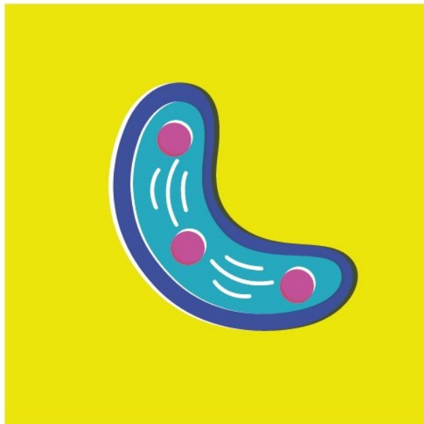
Sin trapping
